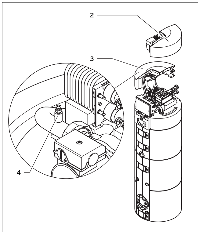
Рис. 6.2 Обезвоздушивание со стороны питьевой воды
