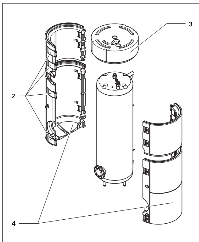
Rys. 5.2 Demontaż izolacji/obudowy
