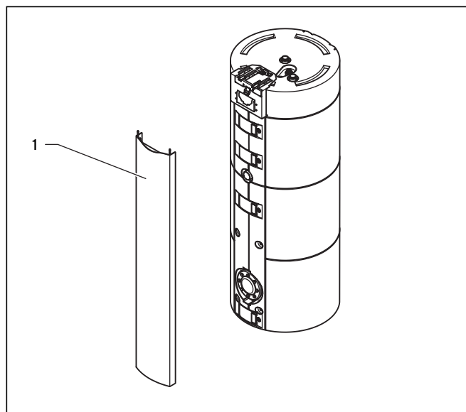
Rys. 5.1 Zdejmowanie drzwi
