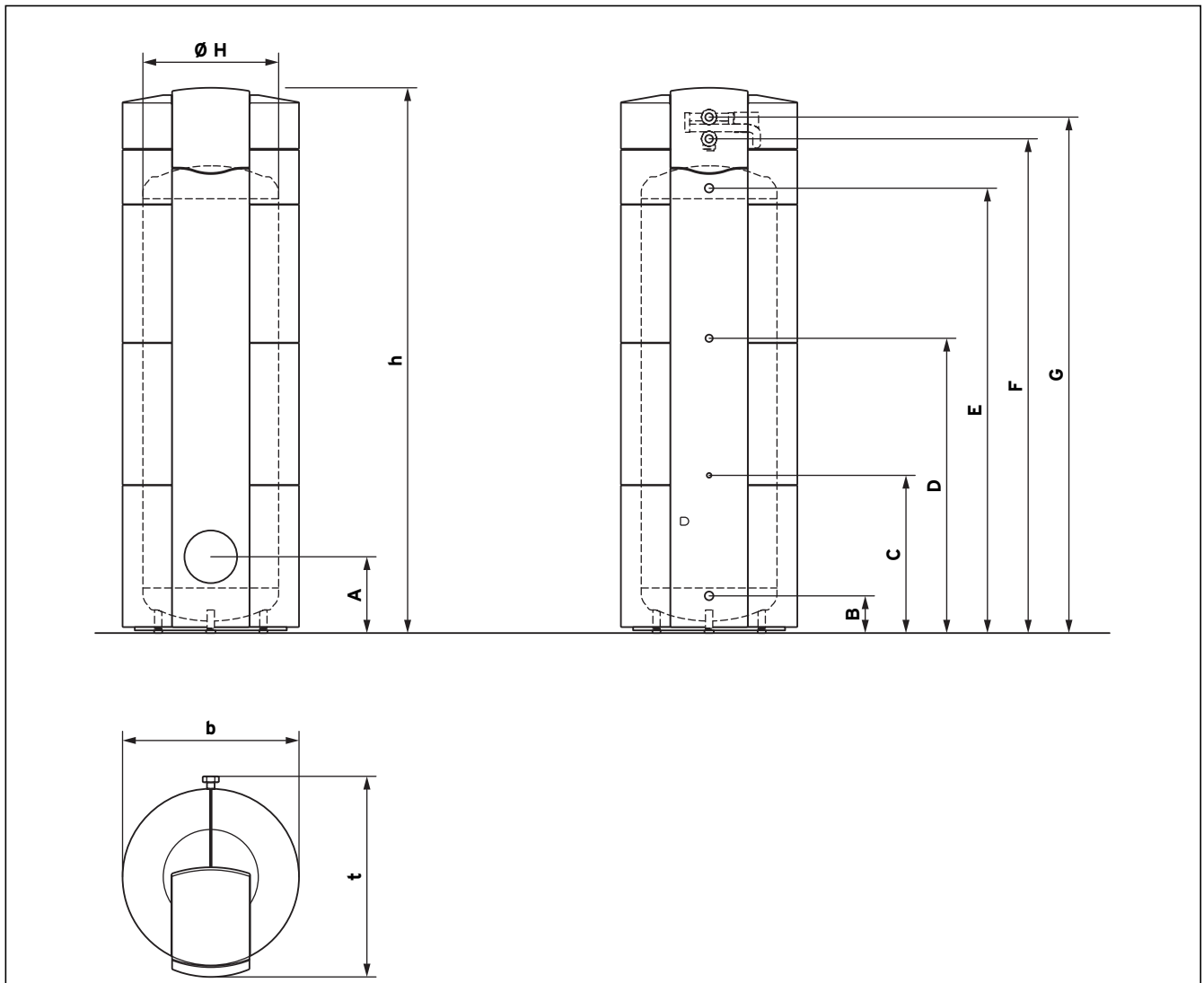
Рис. 5.6 Размеры прибора и подсоединения
