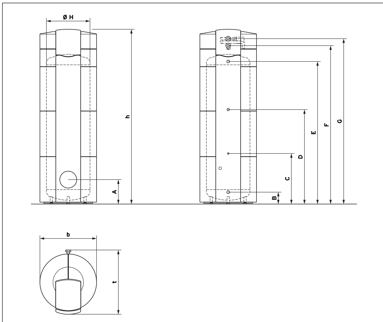
Rys. 5.6 Wymiary urządzenia i przyłączy
