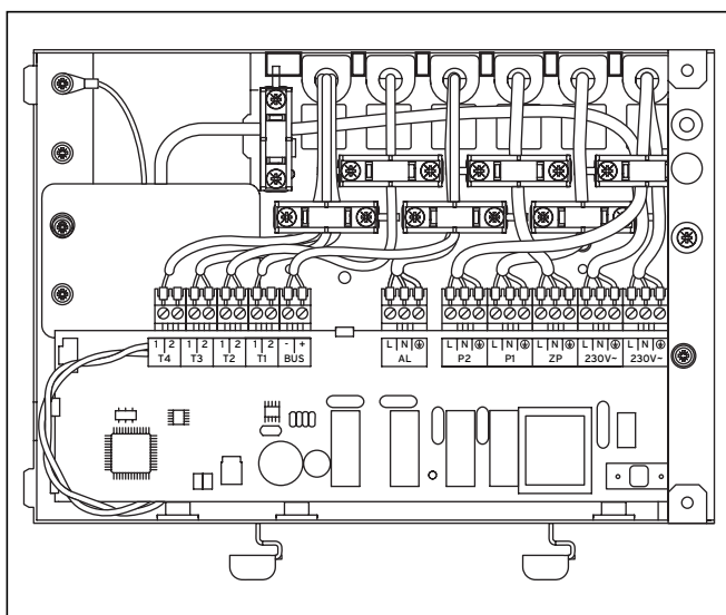
Рис. 5.10 Электроподключения actoSTOR
