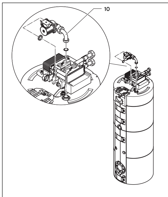
Rys. 5.8 Montaż pompy ładowania ciepłej wody
