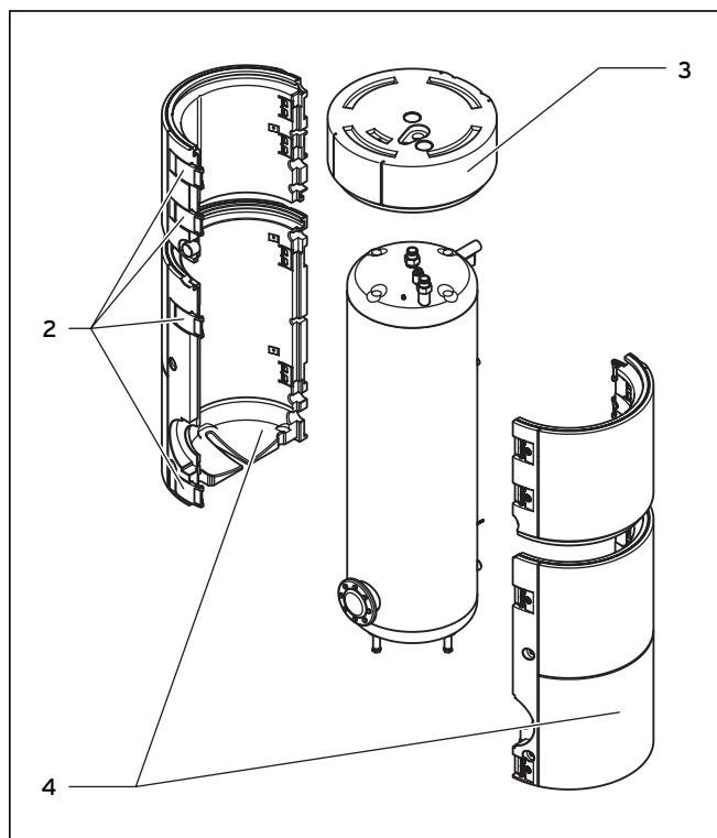
Рис. 5.2 Демонтаж изоляции/обшивки
