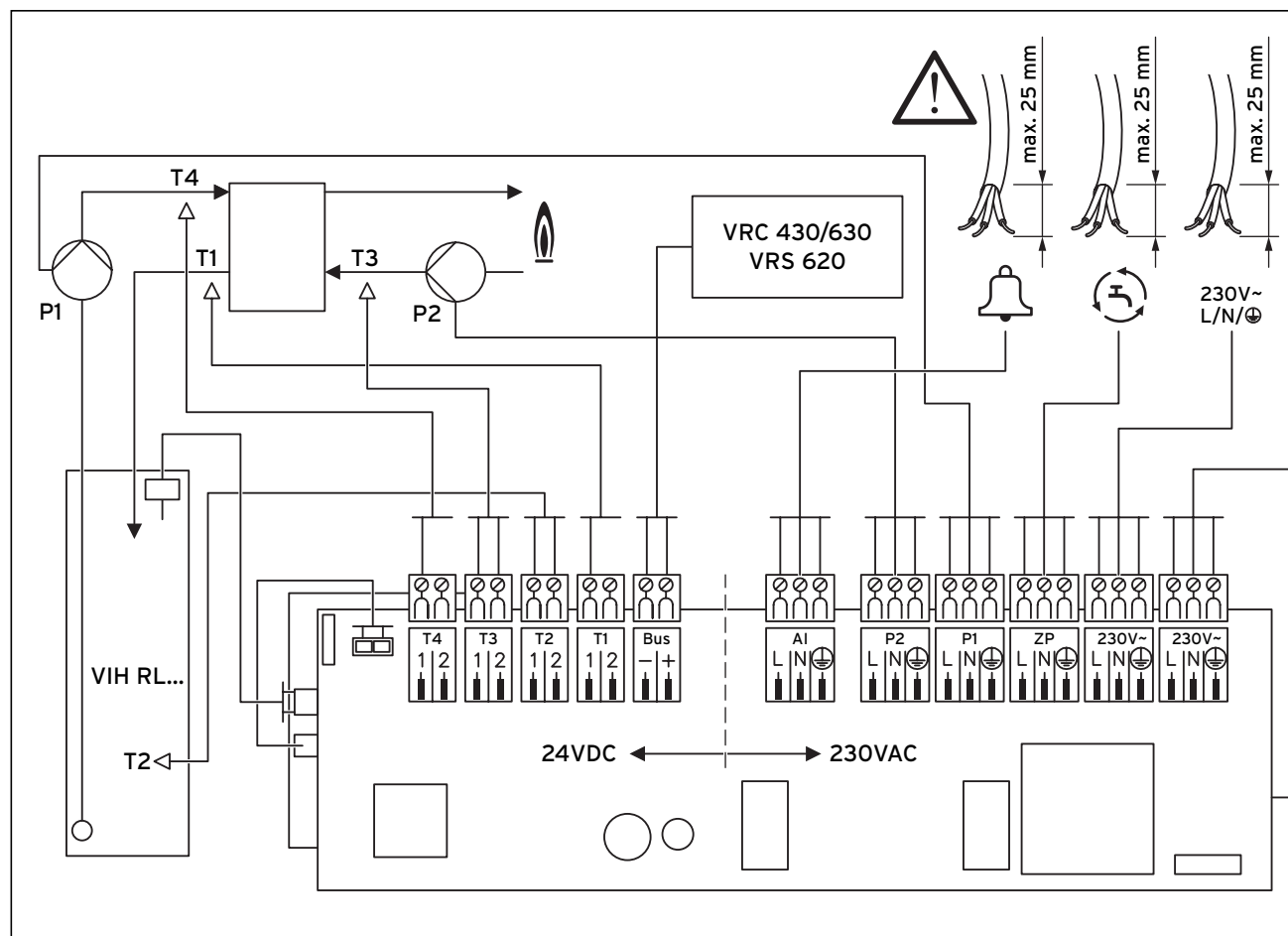
Rys. 5.15 Plan obwodu
