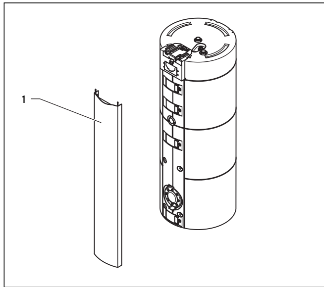
Рис. 5.1 Удаление заслонки
