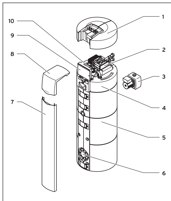
Рис. 2.1 Конструкция actoSTOR
