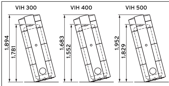
Мал. 5.3 Розміри перекидання actoSTOR
