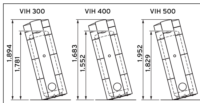
Rys. 5.3 Wymiary actoSTOR po złożeniu
