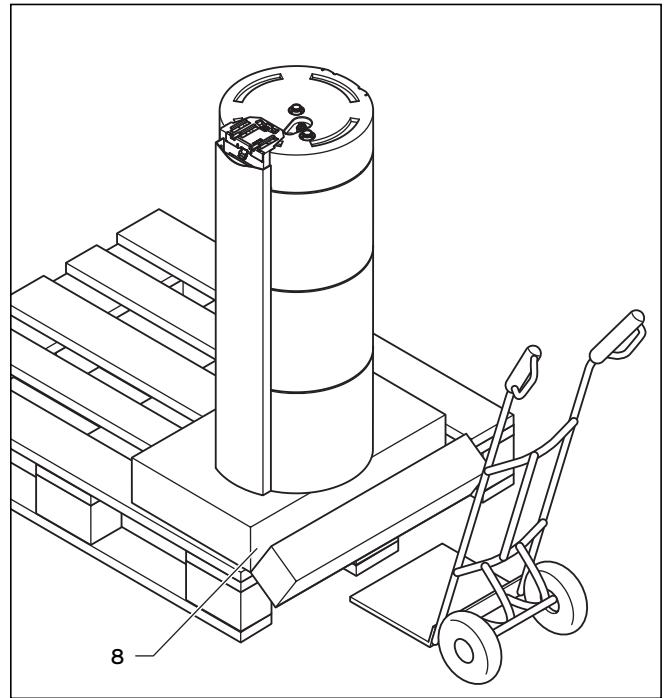
Мал.5.5 Транспортування без транспортної упаковки
