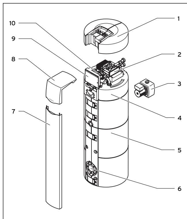
Rys. 2.1 Budowa actoSTOR
